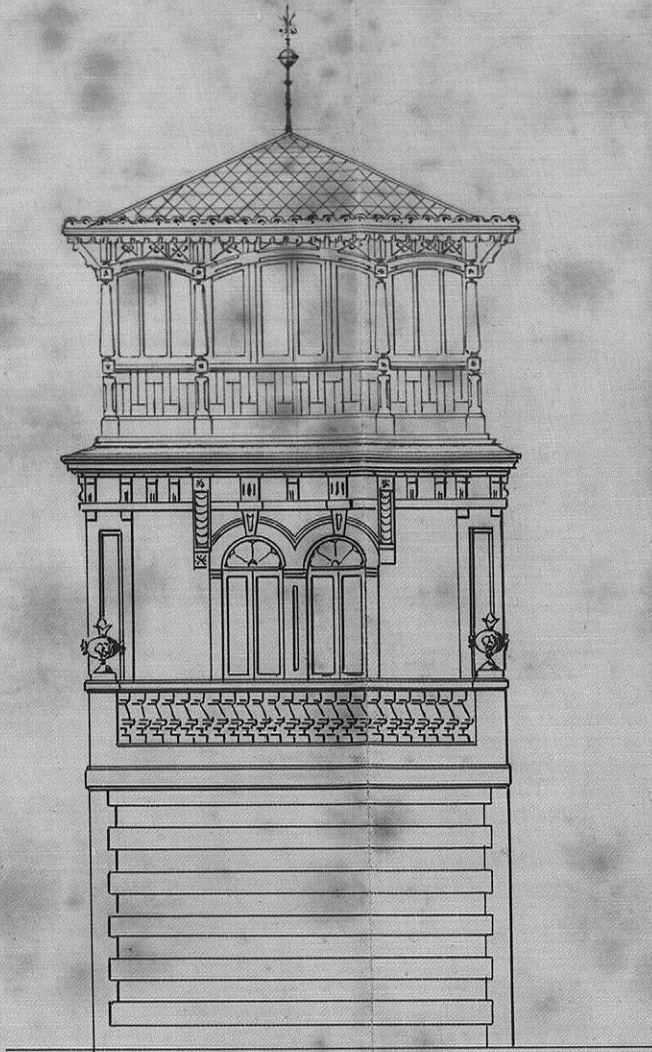
COSTADO
