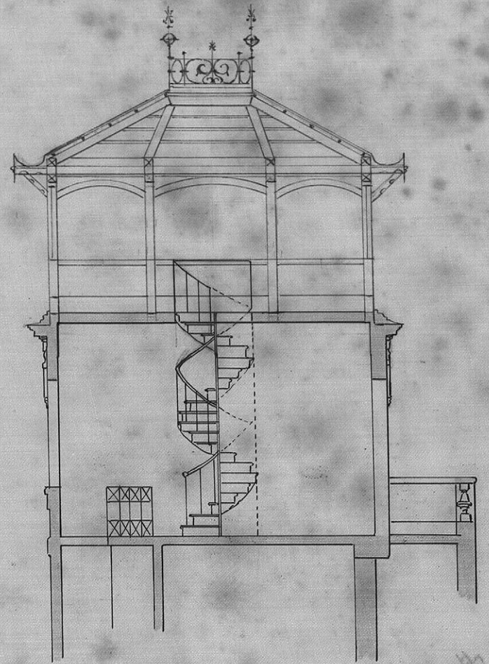
SECCION
