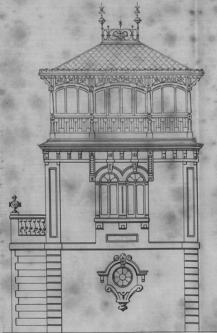
FRENTE
